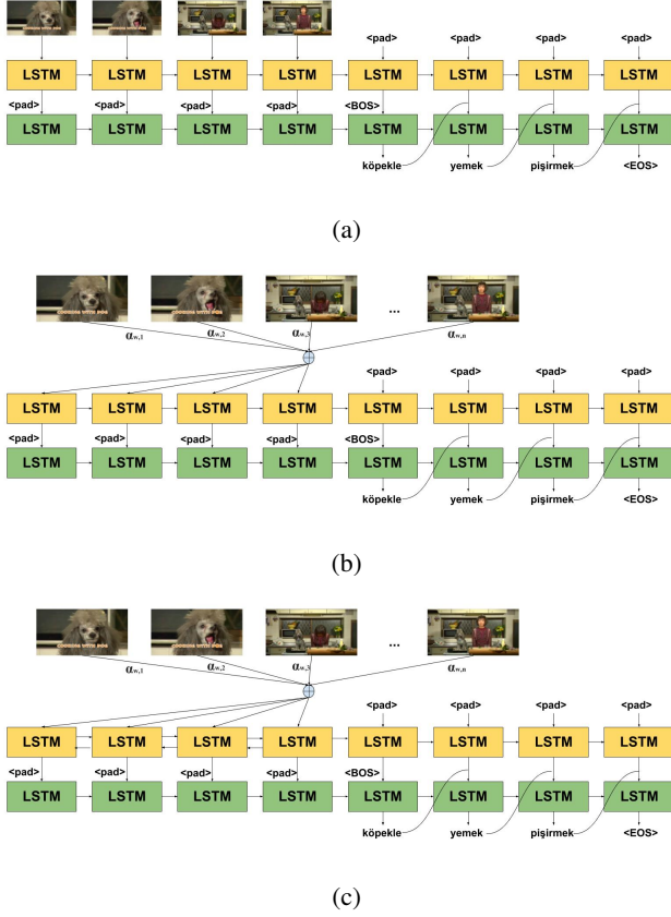
Şekil 1: Gerçekleştirimi yapılan LSTM tabanlı nöral video altyazılama modelleri. (a) Tek yönlü model, (b) Tek yönlü nöral dikkat mekanizması ile donatılmış model, (c) Çift yönlü nöral dikkat mekanizmasına sahip model.
